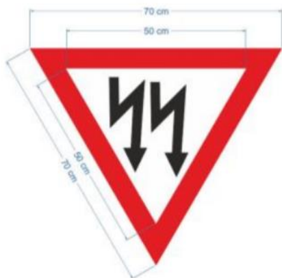
Rys. 6.3. Wymiary znaków kajakowych ostrzegawczych
